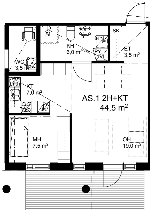
Asunnot 1. kerros A1
